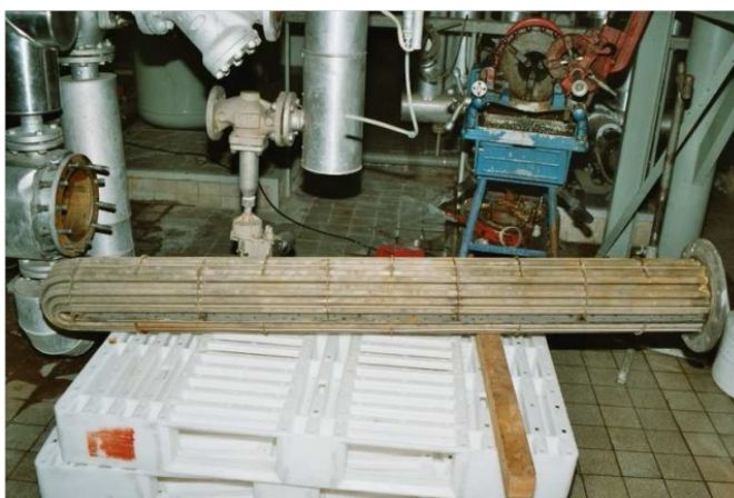
Výměník tepla po demontáži po 5 letech provozu bez jakýchkoli servisních prací. Během této doby výměníkem prošlo asi 360 000 m 3 vody, která se ohřívala na 85°C.
